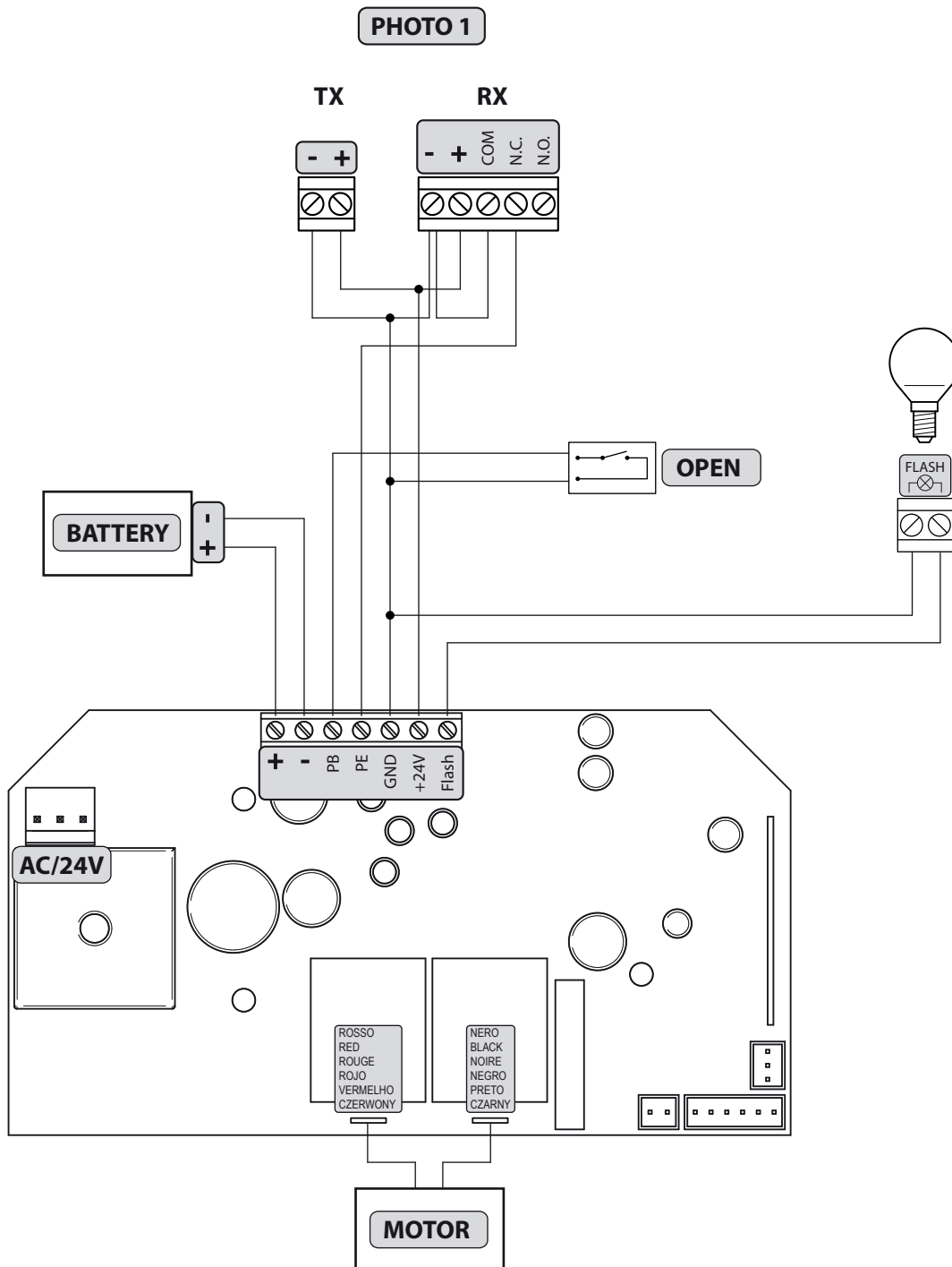
Diagrama de Fiação
