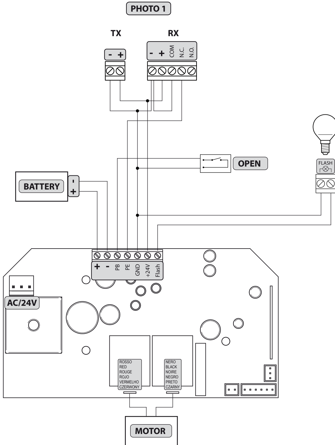
Schéma de câblage
