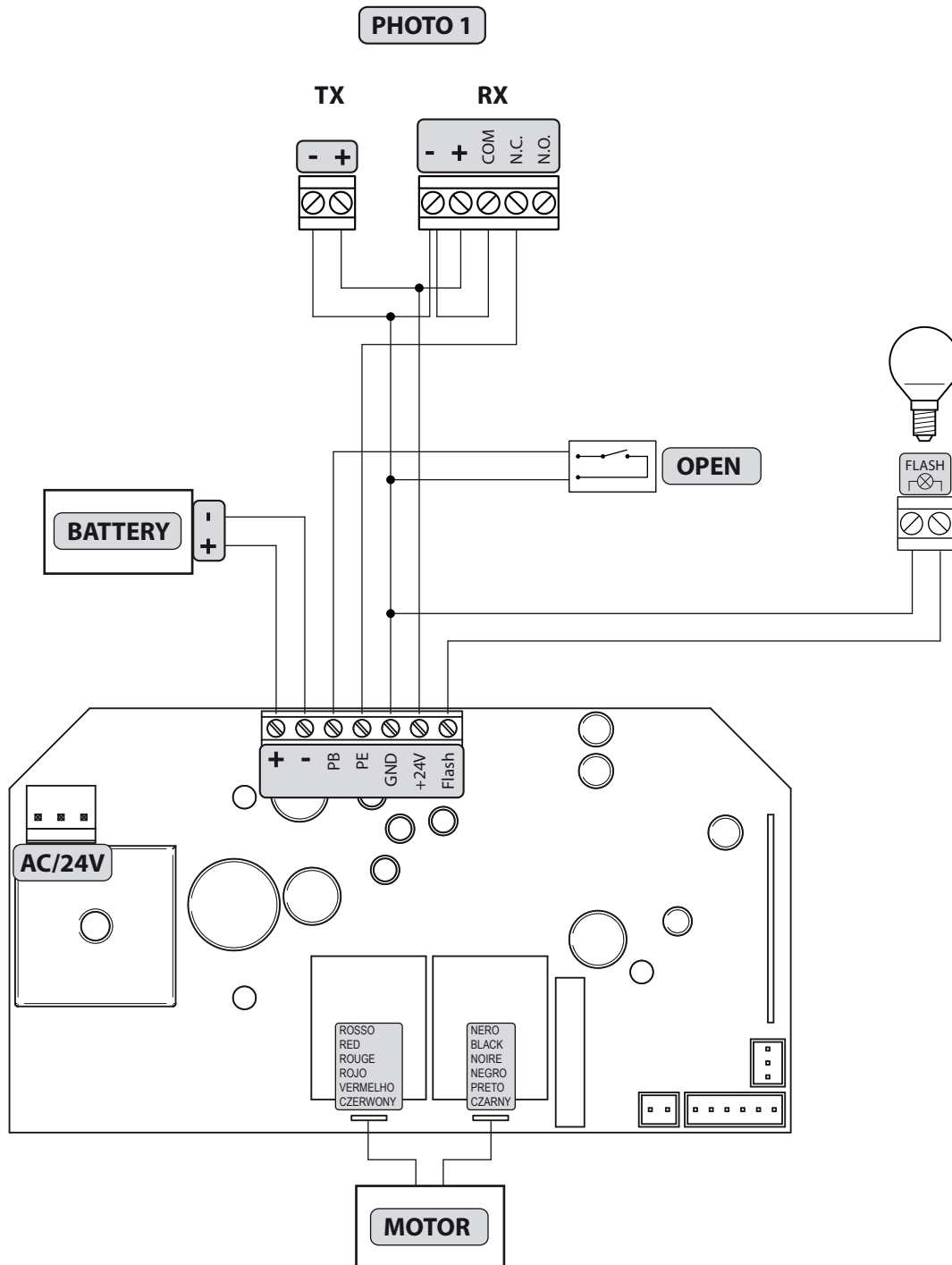
Schemat elektryczny
