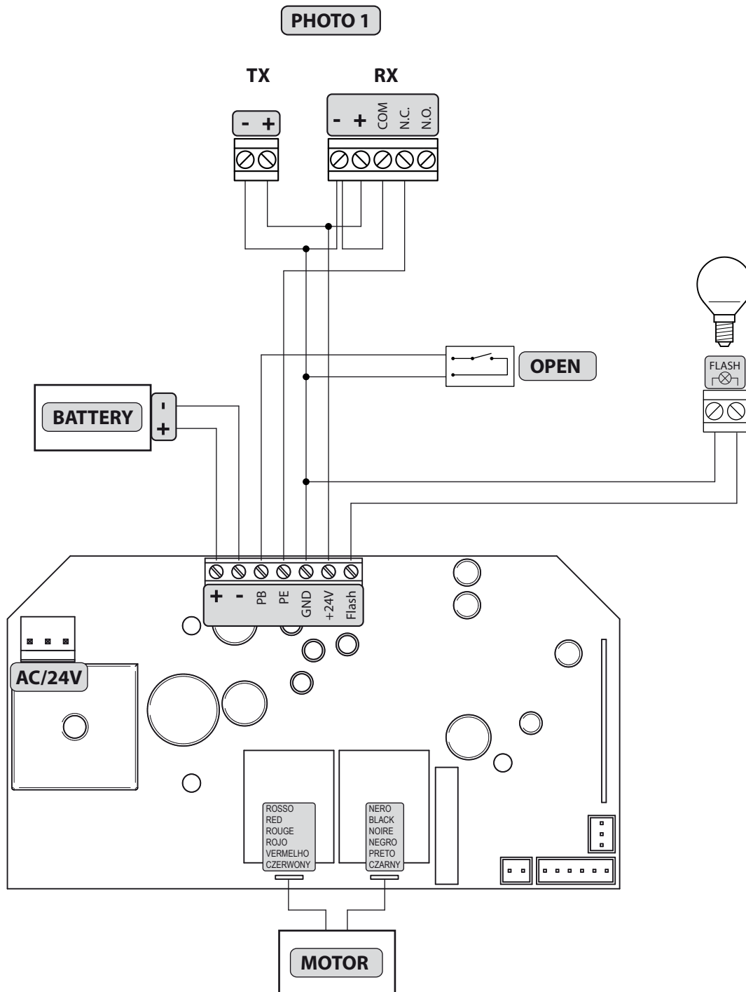
Schema elettrico
