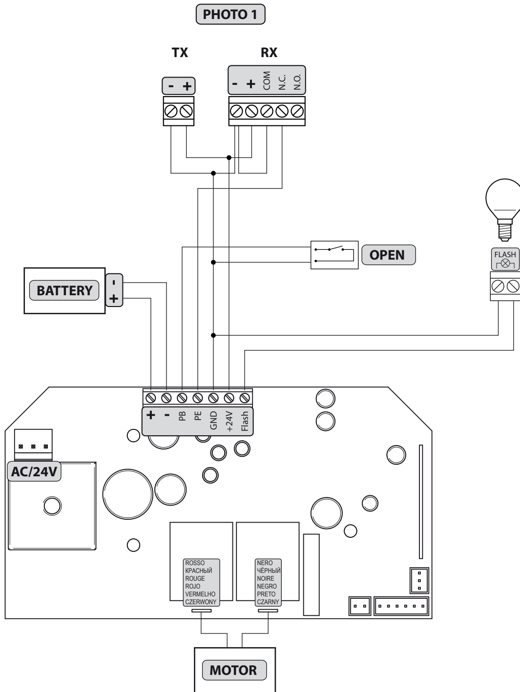
Схема подключения
